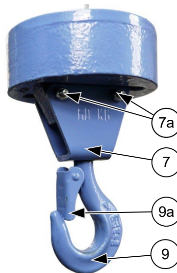
Abb. 65: Drallfänger mit Lasthaken
