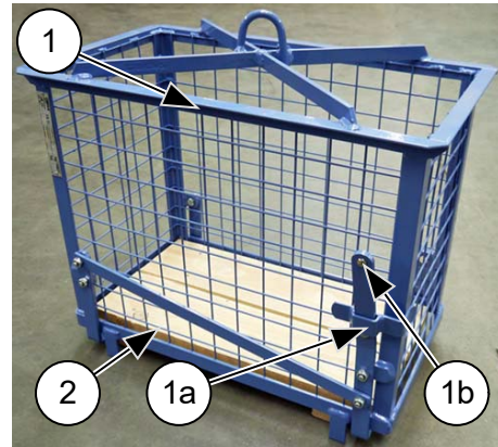
Abb. 32: Steinkorb
