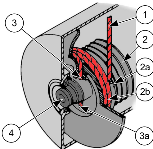
Abb. 62: Drahtseil wechseln 1
