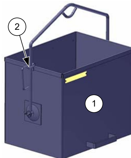
Abb. 30: Kippkübel
