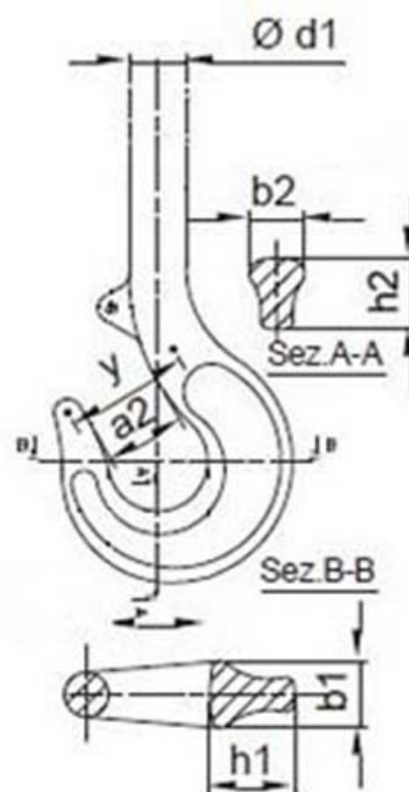
Abb. 66: Verschleiß: Drallfänger mit Lasthaken
