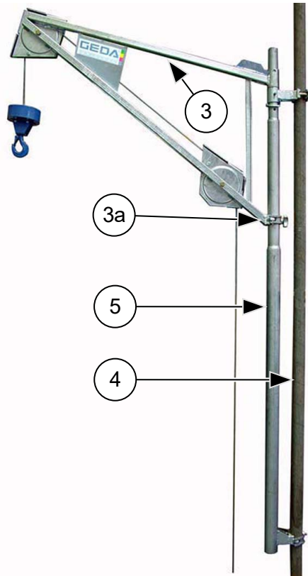
Abb. 41: Einsatz mit Schwenkarmhalterung
