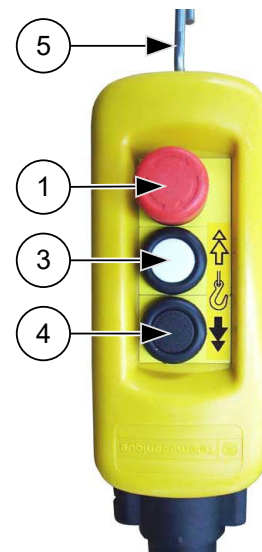
Abb. 53: Handsteuerung 2-stufig
