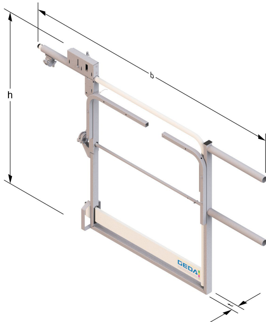
Abb. 18: Etagensicherungstür ECO S
