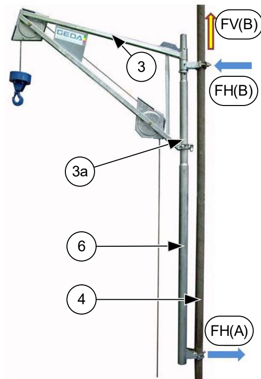
Abb. 42: Universalschwenkarm
