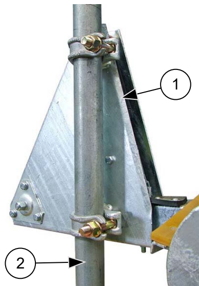
Abb. 38: Winde montieren
