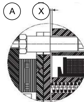
Abb. 61: Motorbremse einstellen (Detail)
