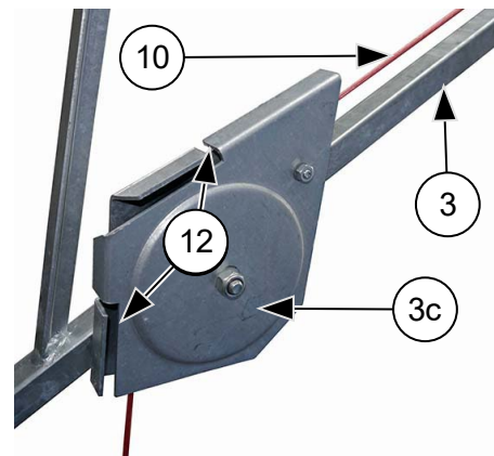
Abb. 51: Drahtseil montieren 2
