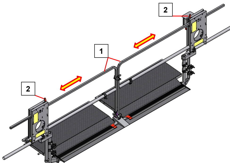
Etagentür 01212 / 01213
