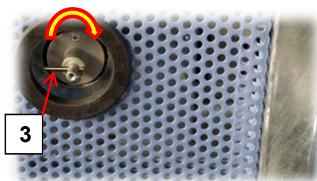
Türschloss entriegelt
