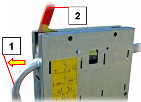
Etagentür 01212 / 01213
